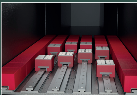
5. Kovametallimodulit asennettuna kulumiselle alttiisiin kohtiin
